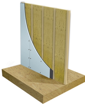
54dB on a stud wall
